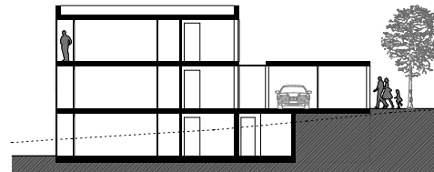
Schnitt Wohnhäuser 1:200
