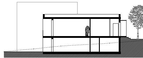
Schnitt Mehrzweckgebäude 1:200
