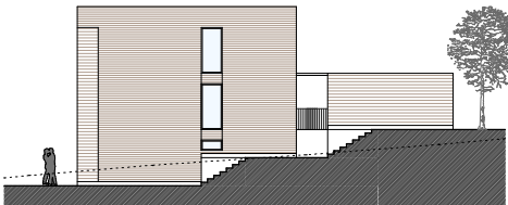
Ost-Fassade 1:200 Wohngebäude
